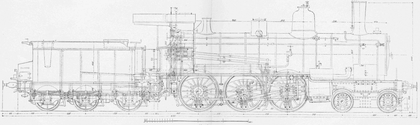
Mastab 1:40. Ansicht der drei- und viercylindrigen Verbund-Schnellzugs-Lokomotiven A 3 T Nr. 201 und 202 samt Tender.
