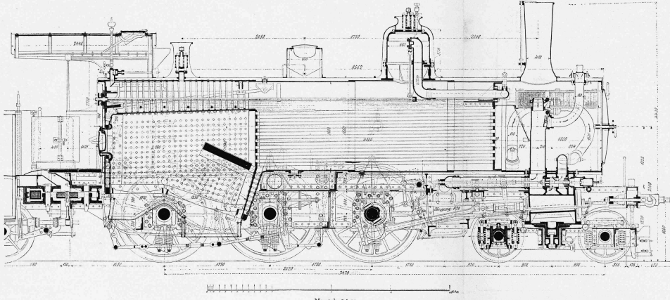
Mastab 1:40. Längenschnitt der viercylindrigen Verbund-Schnellzugs-Lokomotive A 3 T Nr. 202 der Gotthardbahn.
