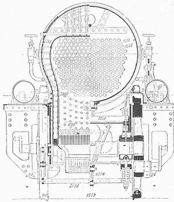
Querschnitt.
