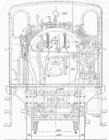
Hinter-Ansicht.
