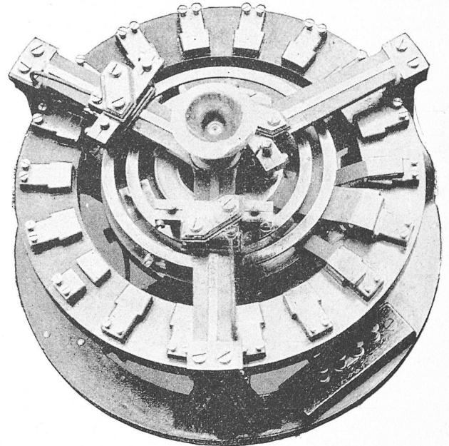
Fig. 10. Verteilungsapparat.
