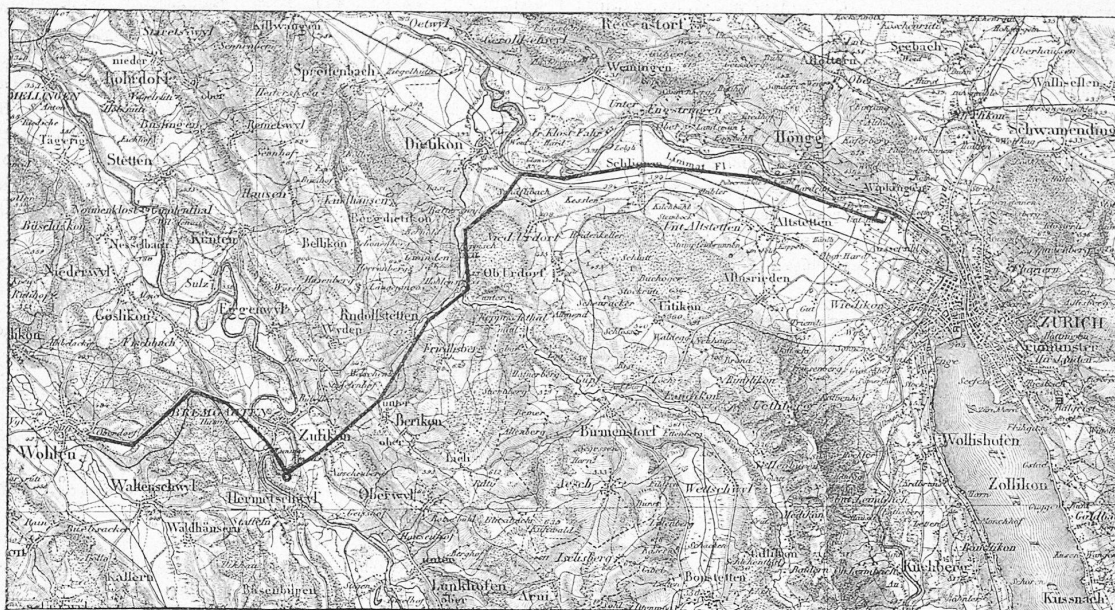
Fig. 10. Leitung von Bremgarten-Zürich nach Wohlen und nach Zürich. Masstab 1:150 000. Unter Benutzung der Dufourkarte mit Genehmigung des eidg. topogr. Bureaus.
