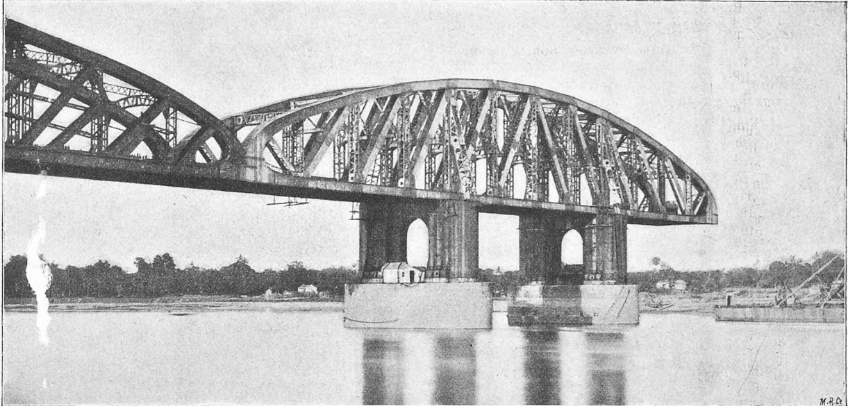
Fig. 5. Cantilever-Träger.
