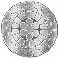
Patentirte „verschlossene“ Drahtseile.
