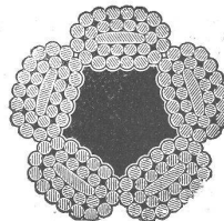
Patentirte „flachflitzige“ Drahtseile.
