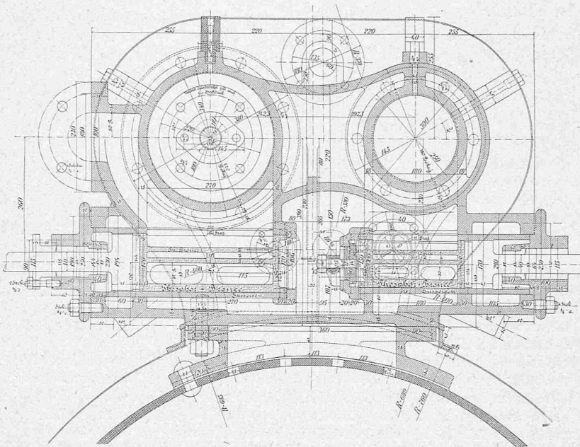
Fig. 4. Schnitt durch die Dampfzylinder. Masstab 1:10.
