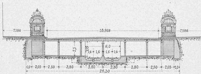
Fig. 8. Querschnitt durch die Station III «Vazsikörút». — Masstab 1:300.
