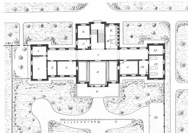
Erdgeschoss-Grundriss 1 : 500.
