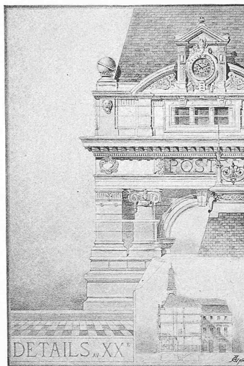
Travée 1 : 160.
