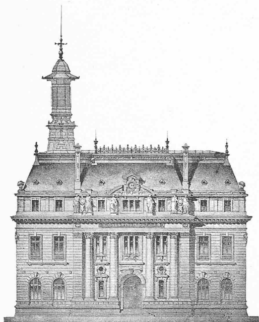
Westfassade 1 : 500.
