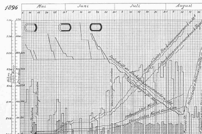
Fig. 9. Foundation der westlichen Hälfte. — Graphische Darstellung.
