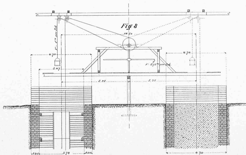
Masstab für Fig. 4—8 = 1:150.
