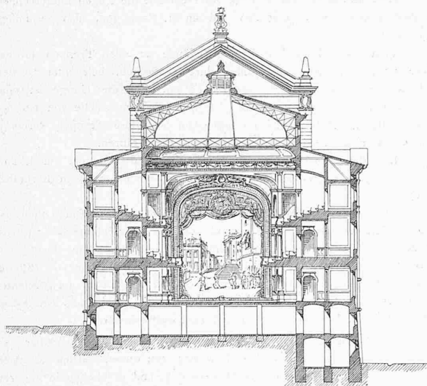
Querschnitt durch das Zuschauerhaus.
