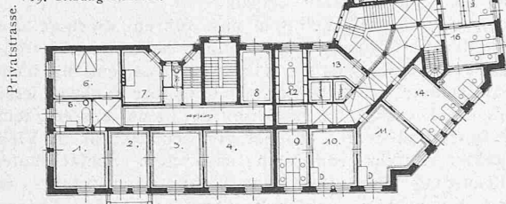
Alfred Escher-Platz. Grundriss vom I. Stock.
