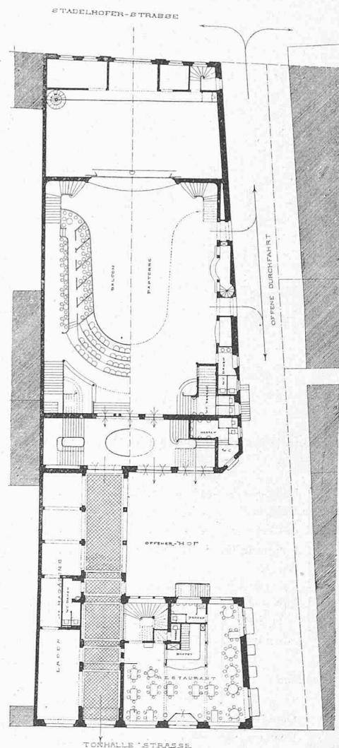
1 : 500. Hauptgrundriss.
