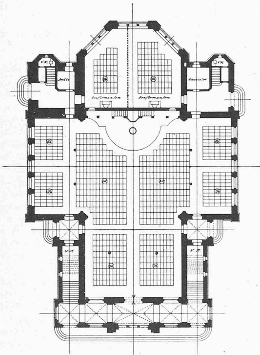
Erdgeschoss-Grundriss.
