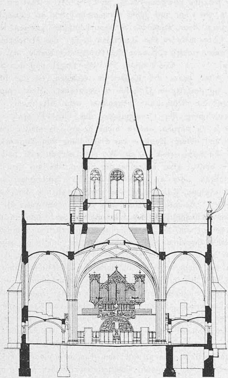
Querschnitt 1 : 500.
