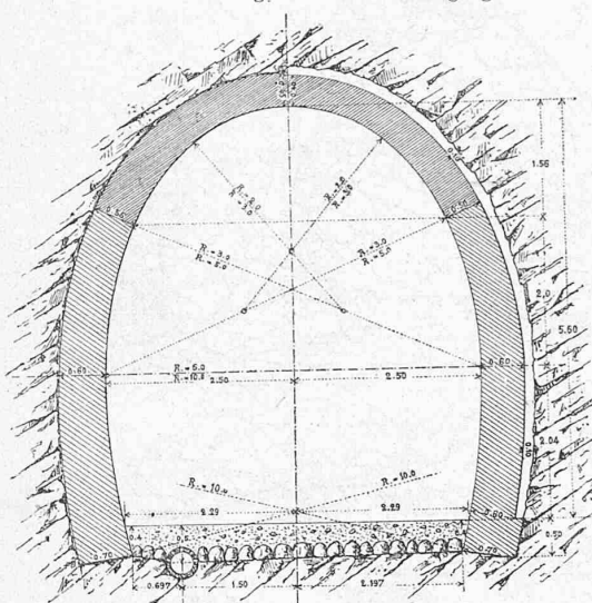
Profil I.
