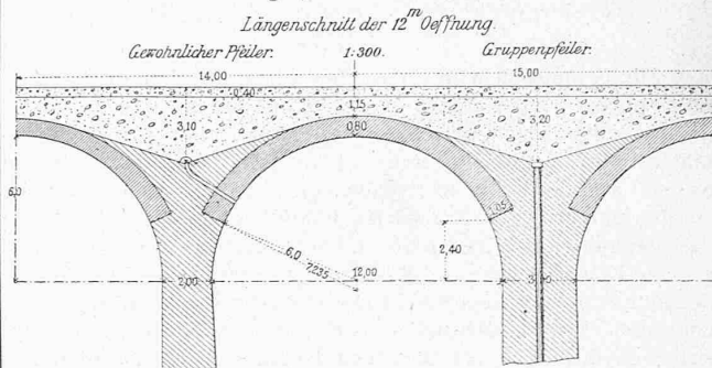
Fig. 4. Lorze-Viadukt.
