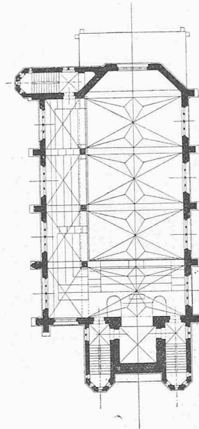
Emporen-Grundriss.
