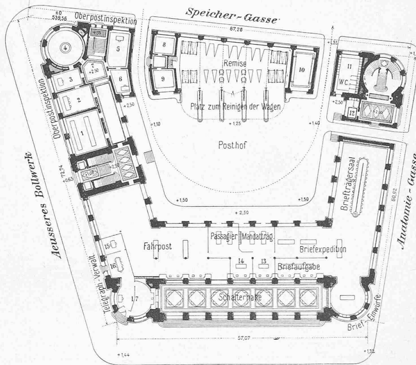
Erdgeschoss-Grundriss 1 : 800.
