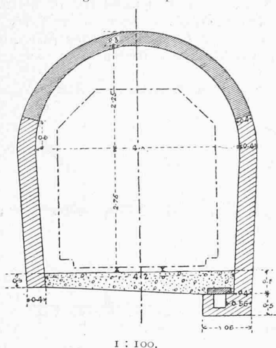
Fig. 1. Tunnelprofil.
