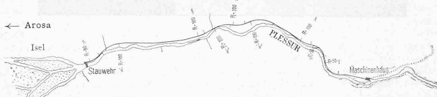
Fig. 3. Situation der Rohrleitung 1:12000.
