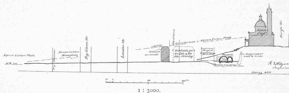
Projekt H_I — Schnitt a—b.
