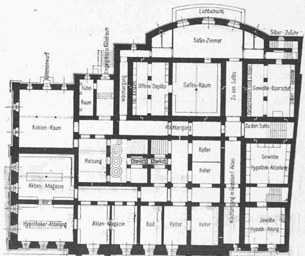
Grundriss vom Untergeschoss 1 : 500.
