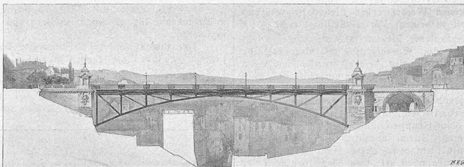
Ansicht 1 : 1000.
