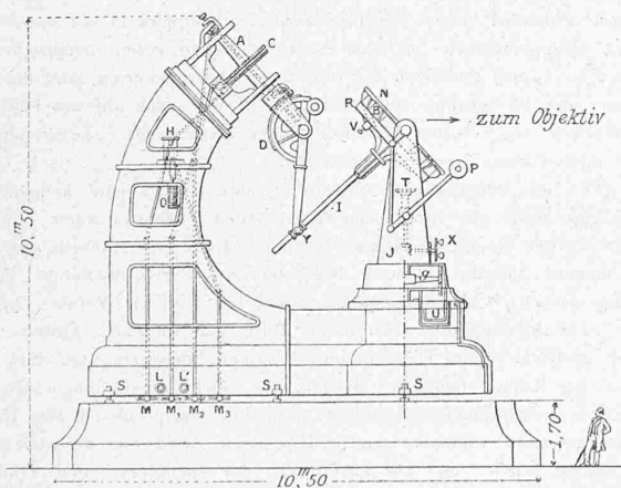
Fig. 1. Siderostat.
