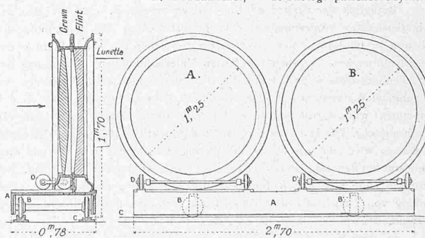
Fig. 3. Anordnung der Objektive.
