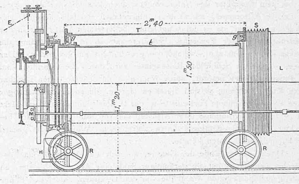
Fig. 2. Seitenansicht des Okulars.
