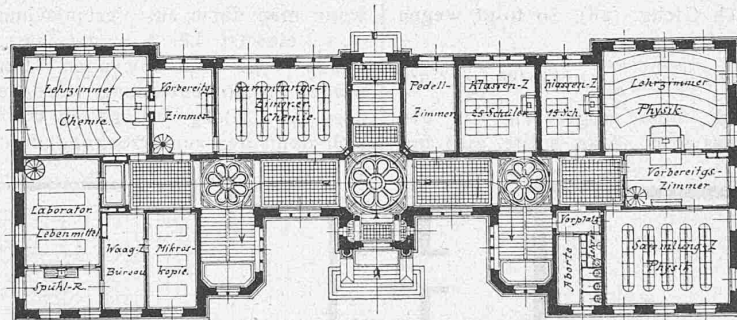
Erdgeschoss-Grundriss 1 : 500.
