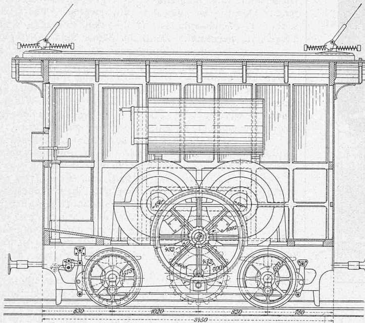
Fig. 24. Längsschnitt.
