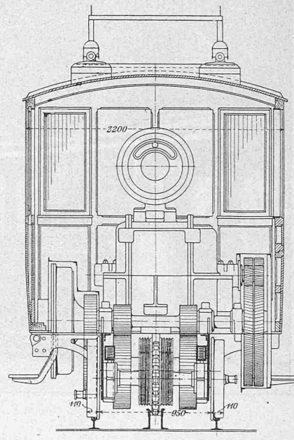
Fig. 26. Querschnitt.
