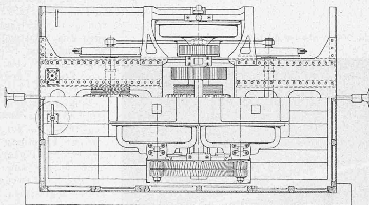
Fig. 25. Grundriss.
