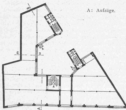
Fig. 7. Erdgeschoss-Grundriss 1:800.
