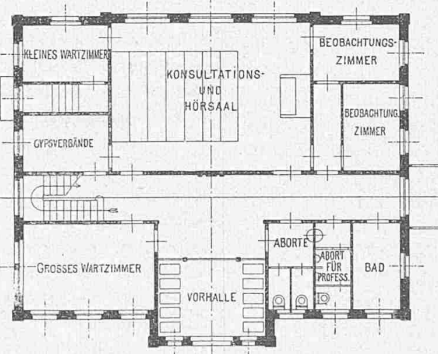
Grundriss vom Erdgeschoss. 1: 300.
