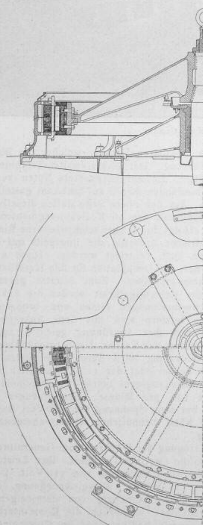
Fig. 7. Zweiphasen-Wechselstrom-Generator von 1200 P. S.
