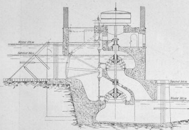
Fig. 5. Turbinenanlage älterer Ausführung. 1:300.
