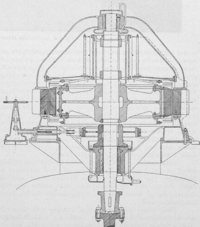
Fig. 8. Gleichstrom-Generator von 1200 P. S.
