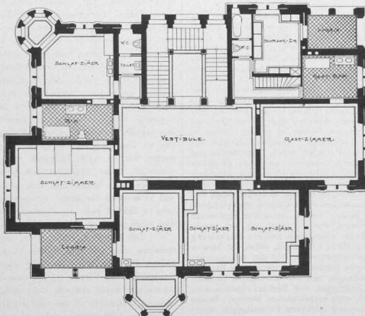
Grandriss vom I. Stock. 1:250.
