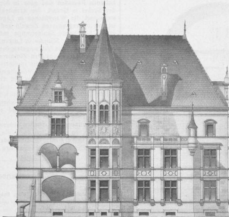
Ostfassade 1:250.
