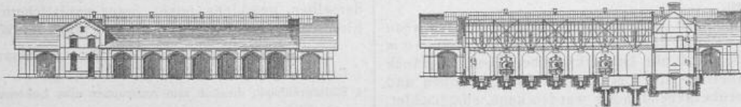
Fig. 6. Seitenansicht der Remise. 1:1000.
