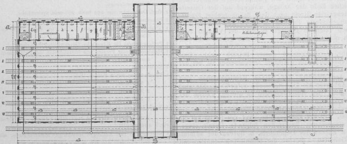
Fig. 8. Grundriss. 1:1000.
