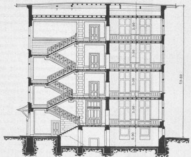
Schnitt C-D. 1 : 300.
