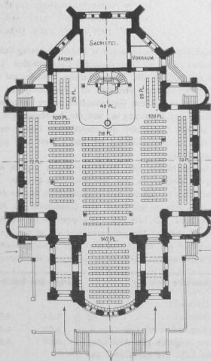
Erdgeschoss-Grundriss 1 : 500.
