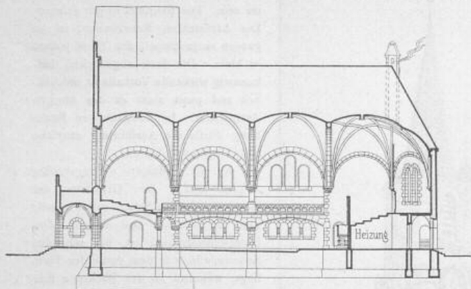
Längenschnitt 1:500.
