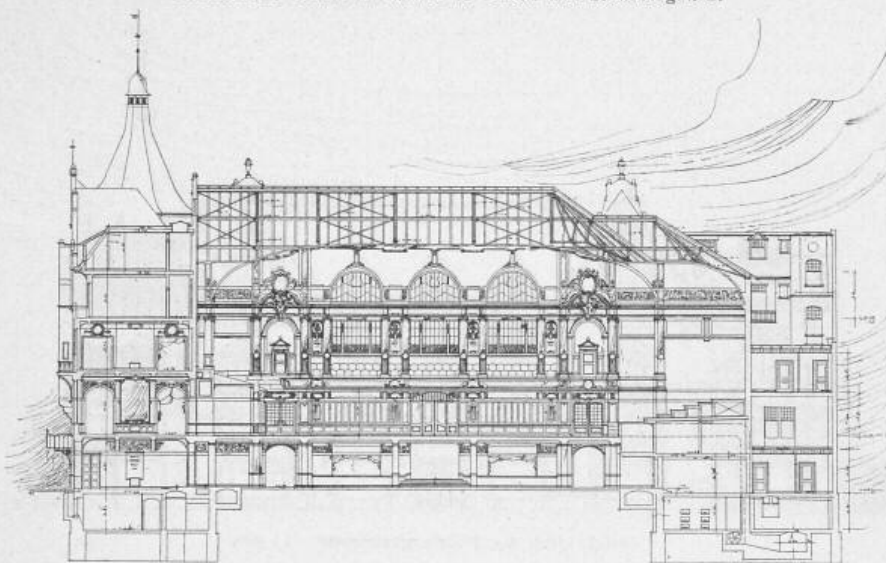
Längenschnitt 1:500.
