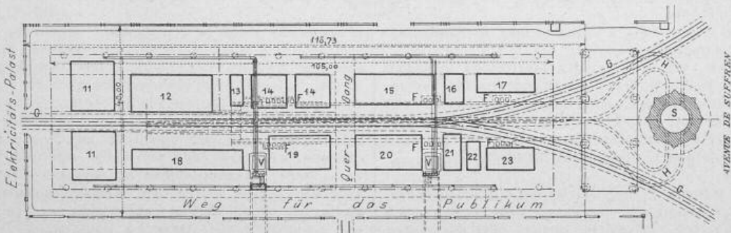
Fig. 3. Grundriss des Kesselhauses «Av. de Suffren». 1:1000.
