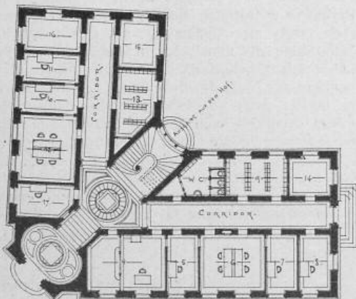
Erdgeschoss-Grundriss.
