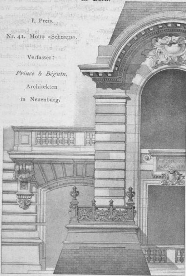
Fassaden-Detail des Eckbaus 1:100.
