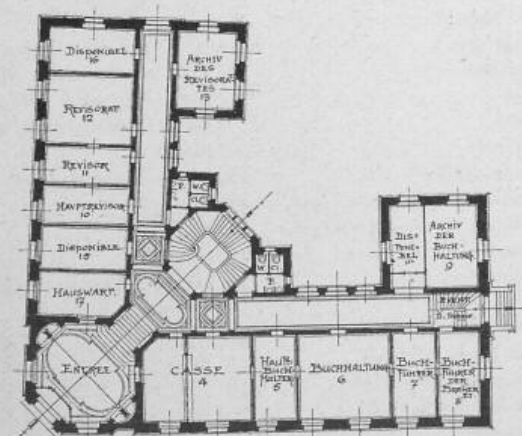
Erdgeschoss-Grundriss.
