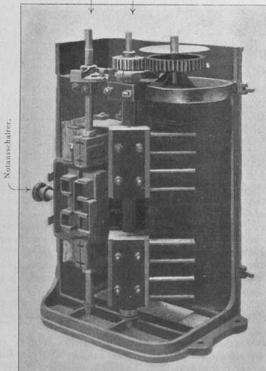
Fig. 32. Controller.
