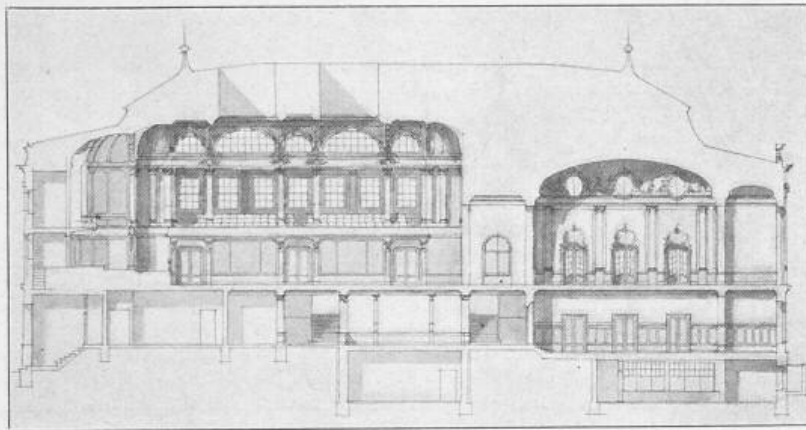
Längenschnitt 1 : 500.
