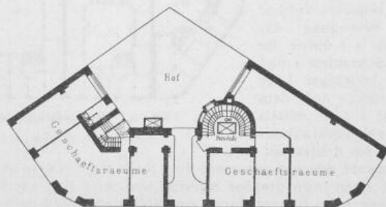
Fig. 36. Kaufhaus Köln. Erdgeschoss 1:500.
