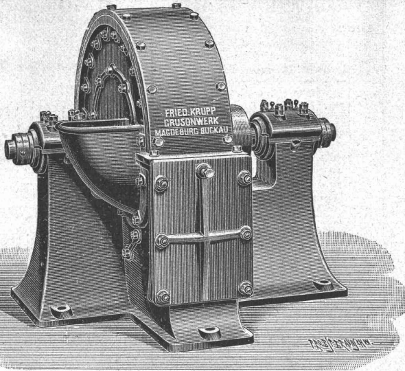
Schlagkreuzmühle.
