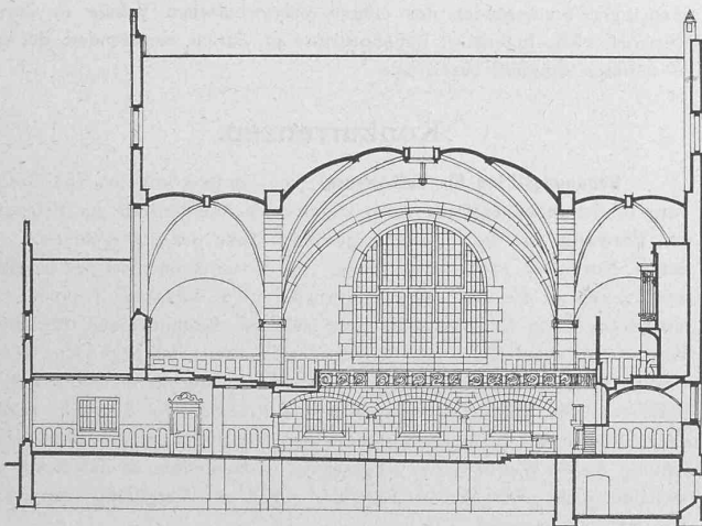
Längsschnitt 1:400.
