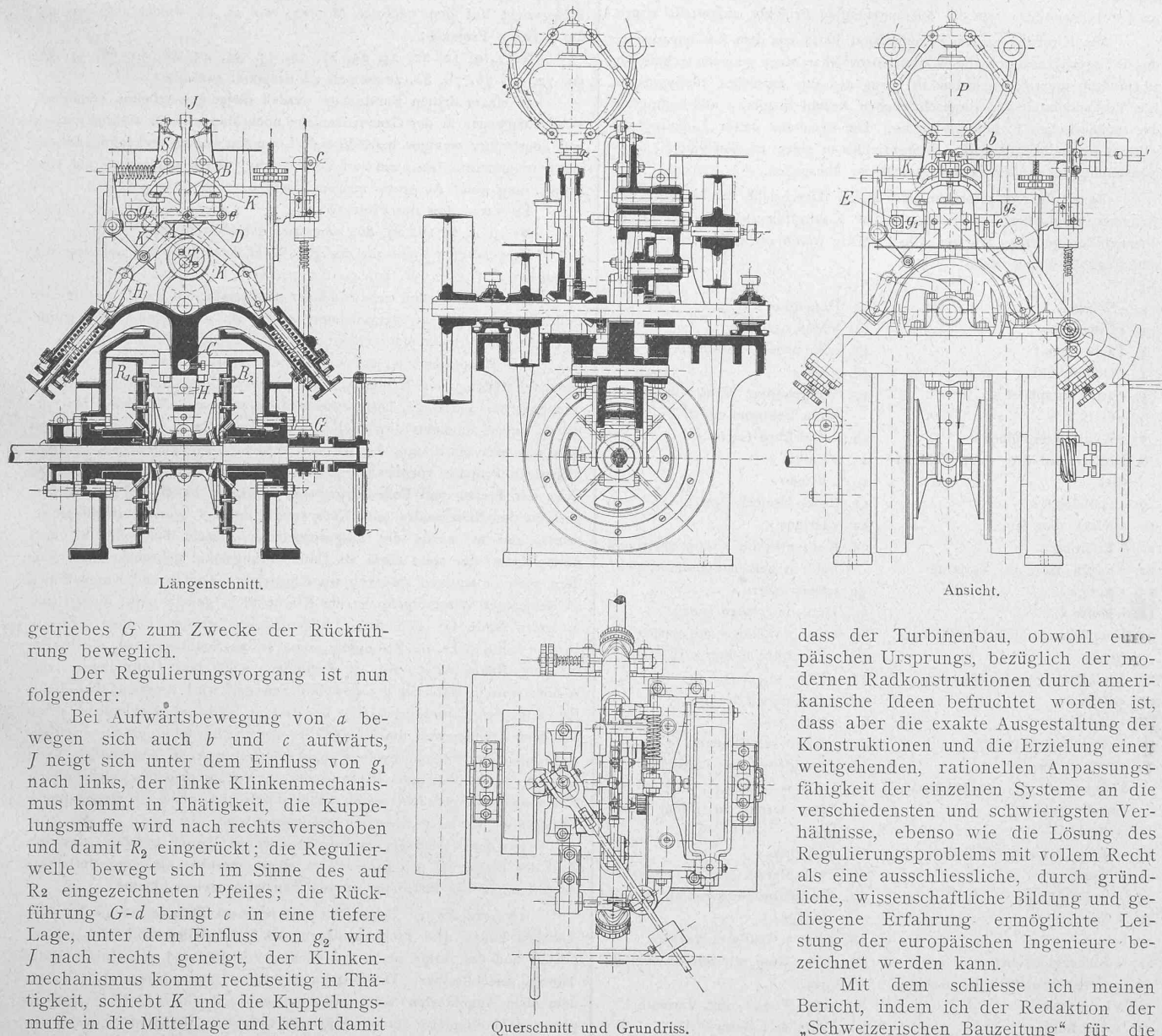
Fig. 70. Klinkenregulator mit Friktionskupplung. — Masstab 1:15.
