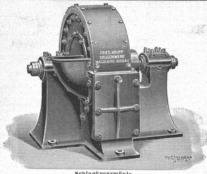
Schlagkreuzmühle.
