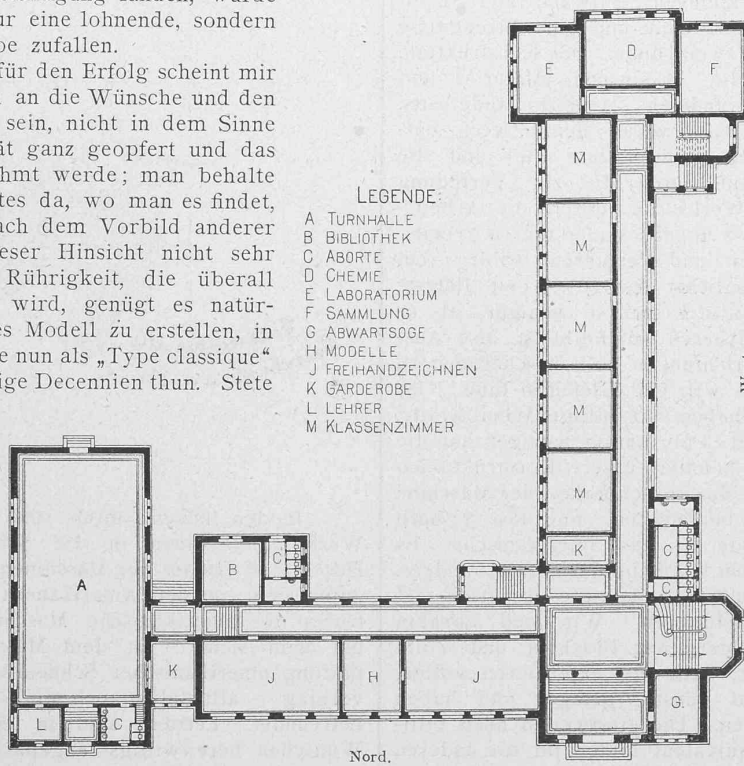
Nord. Grundriss vom Erdgeschoss. Masstab 1 : 750.
