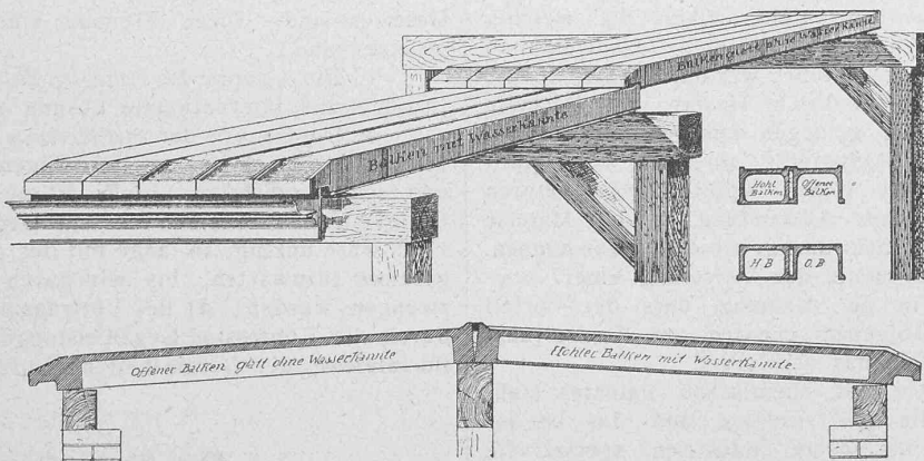
Fig. 8. Wasserdichte Terrassenbalcken — nach unten offen oder geschlossen.
