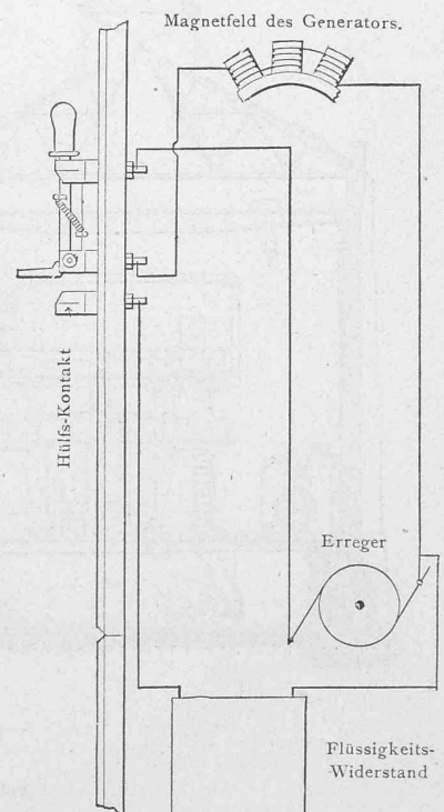
Abb. 7. Erregerschaltung.
