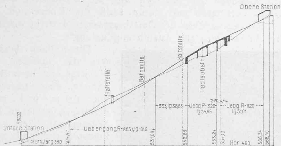
Abb. 2. Längsprofil.
