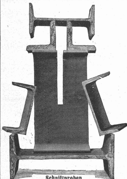
Schnittproben
