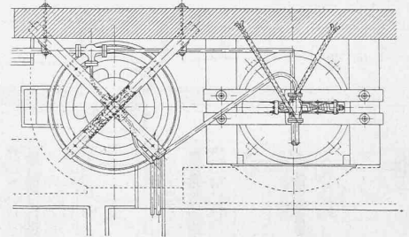
Abb. 65. Die Gewichtsassumulatoren-Anlage. Masstab 1 : 100.
